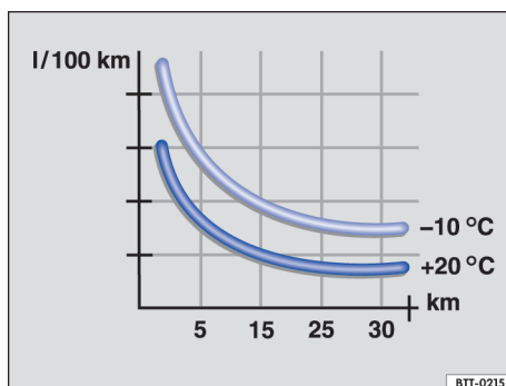
图 78 两种不同环境温度时的百公里油耗（l/100km）。
