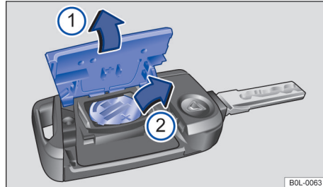
图 40 车辆钥匙：更换纽扣电池
