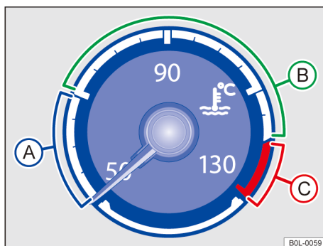
图 14 组合仪表中的发动机冷却液温度表
