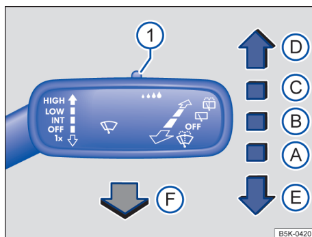
图 67 转向柱右侧：前风窗刮水器操纵杆操作位置
