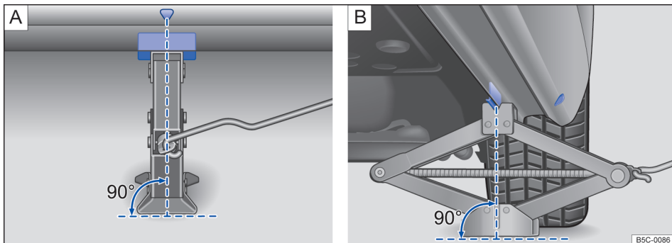
图 147 千斤顶放置在车辆左侧后部
