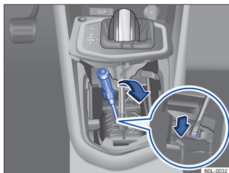
图 87 手动开启变速杆锁
