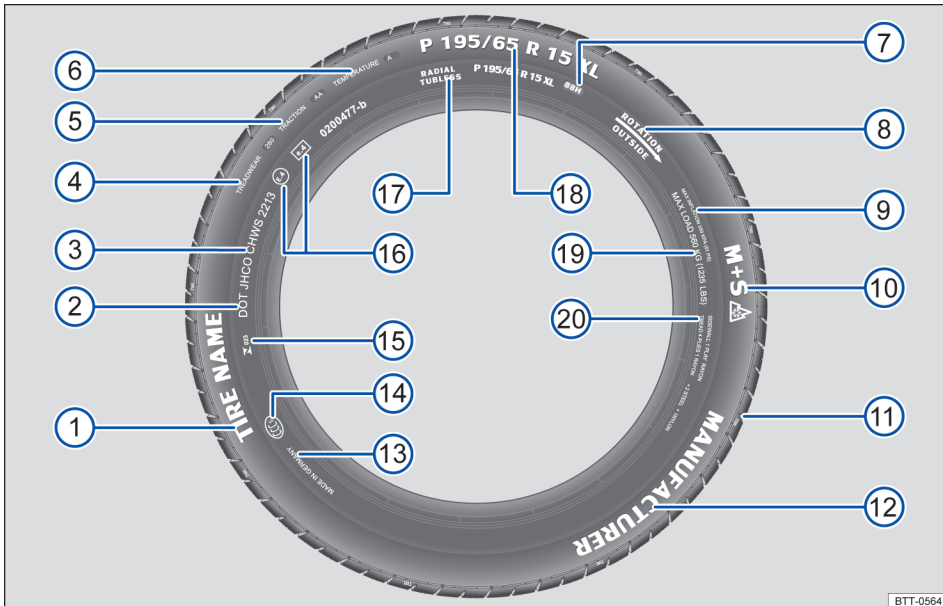
图 142 国际通用轮胎识别字码
