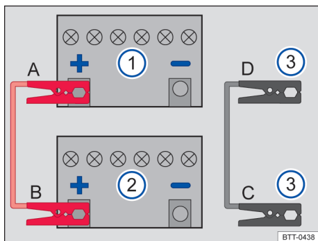
图 120 连接起动辅助电缆的示意图
