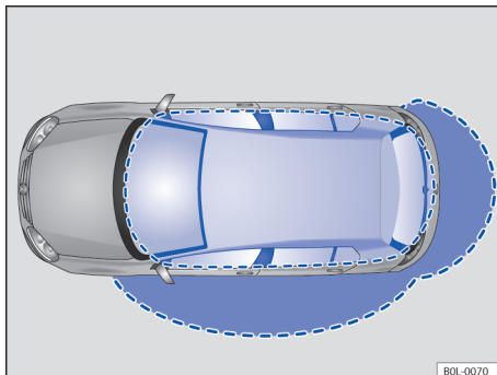
图 41 Keyless Access 闭锁/启动系统：接近范围
