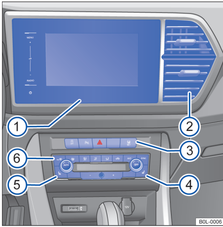
图 6 中控台上部概貌
