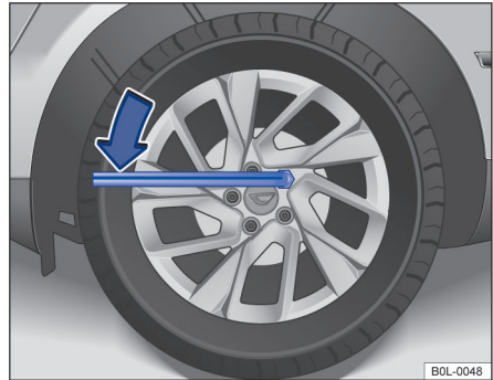
图 145 更换车轮：拧松车轮螺栓
