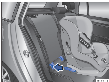
图 36 示意图: 利用固定臂安装 ISOFIX 儿童座椅
